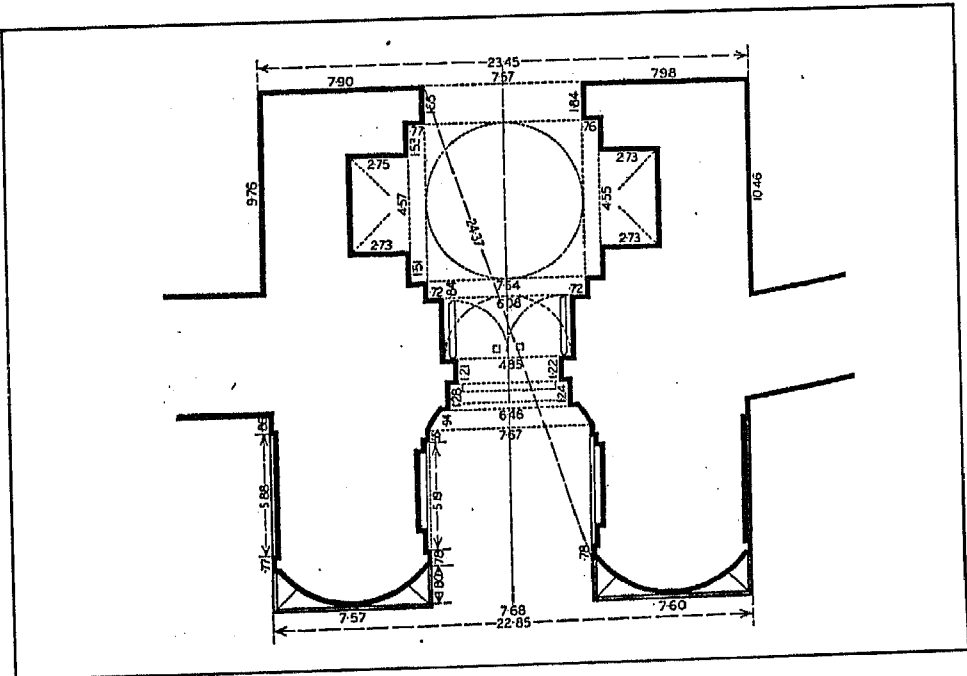
شكل (١٢) باب الفتوح، مسقط أفقى عن كزيويل
